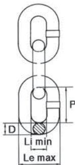
Rundstahlketten GK 10, Sondergüte, PAS 1061
